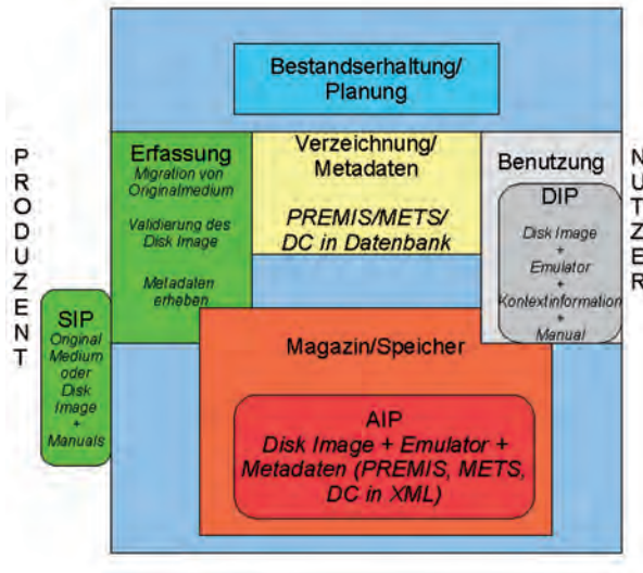
Abbildung 1: OAIS-Funktionsmodell
